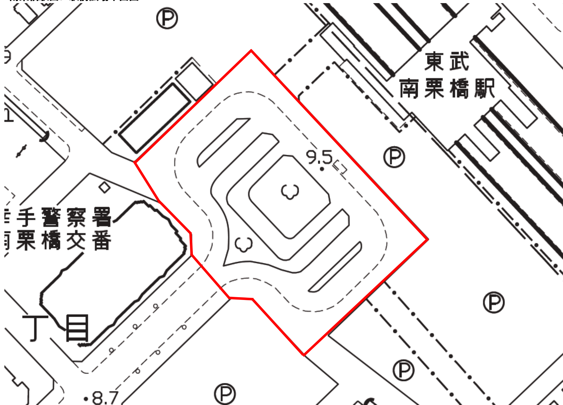
南栗橋駅西口駅前広場平面図
