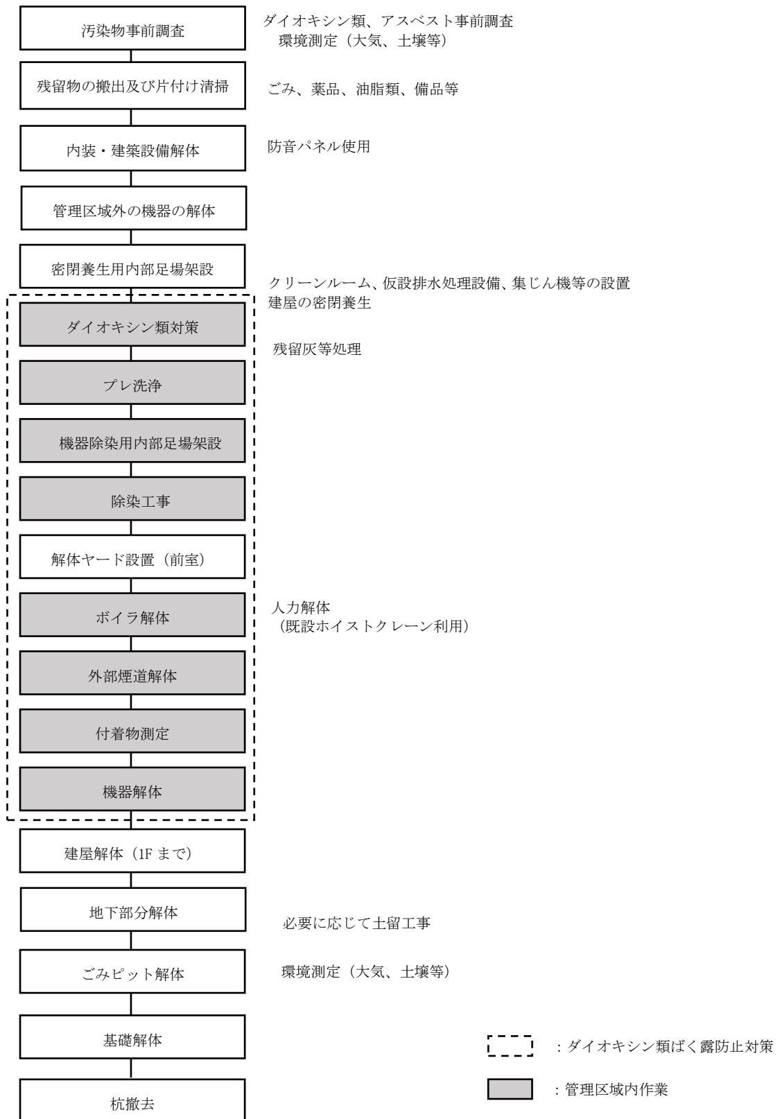
図-5-1 解体工事手順（参考）
