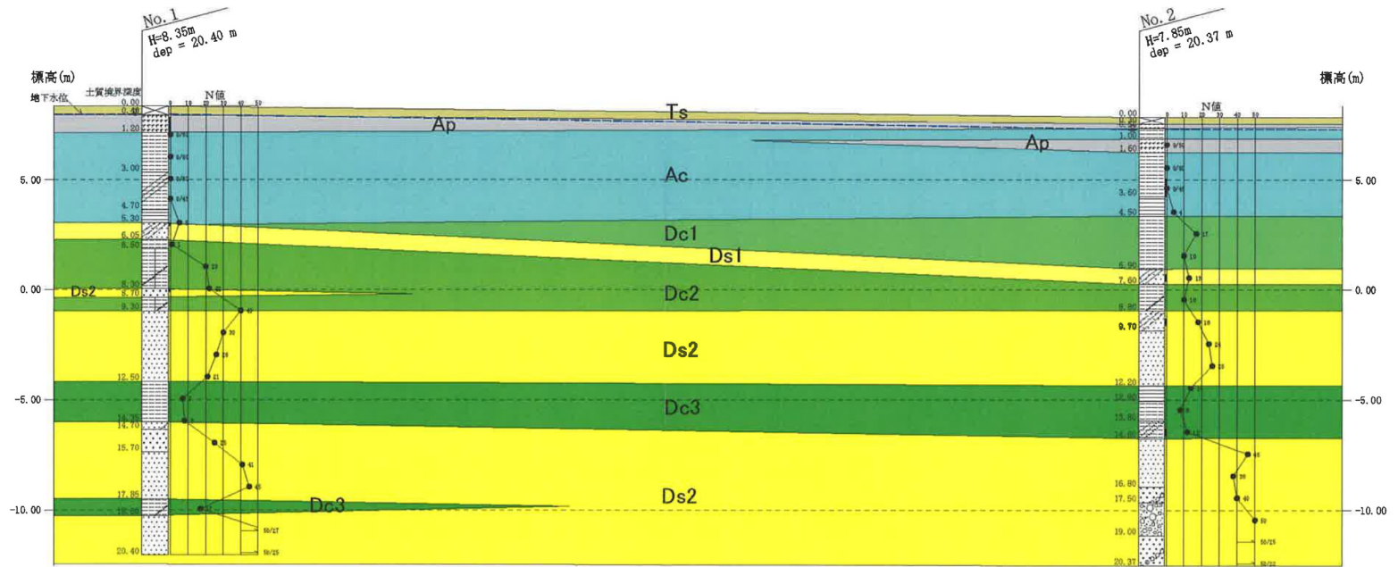
地質想定断面図 (参考)
