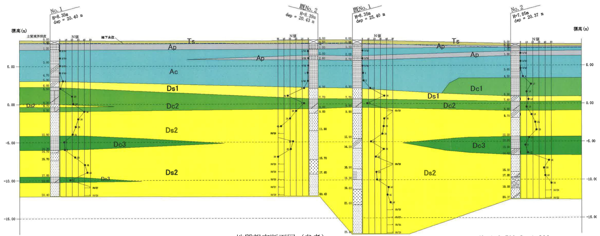
地質想定断面図 (参考)
